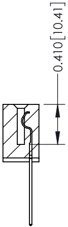
SECTION A-A
