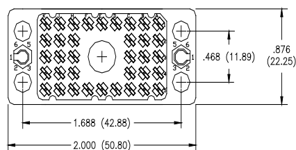
36 PIN RECEPTACLE
