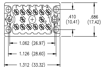
36 PIN RECEPTACLE
