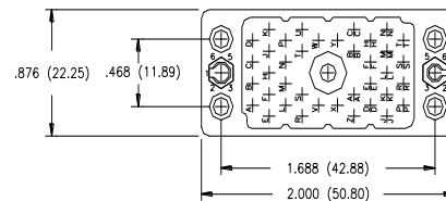
38 PIN RECEPTACLE
