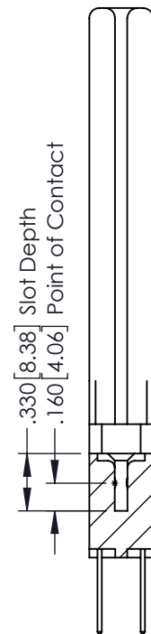
SECTION A-A
