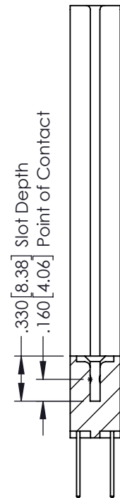
SECTION A-A
