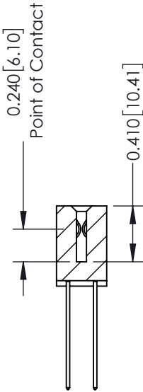
SECTION A-A
