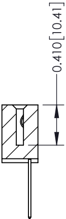
SECTION A-A
