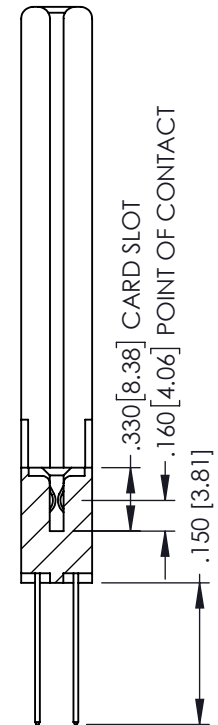
SECTION A-A
