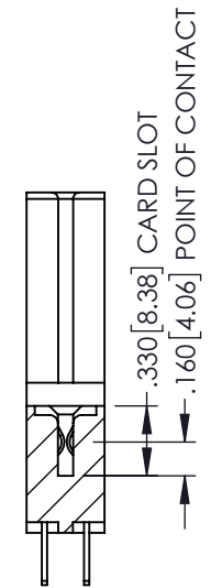
SECTION A-A
