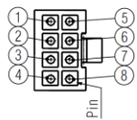
Steckerbelegung/ Connector connection
