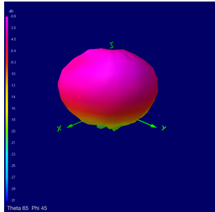
5700 MHz
