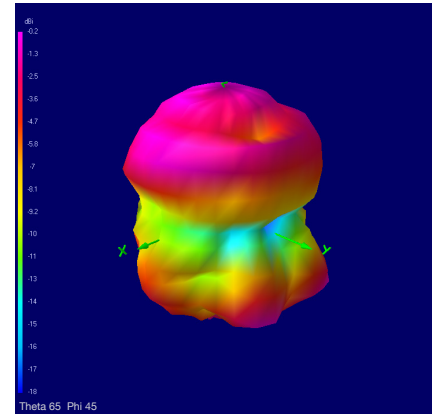
3600 MHz
