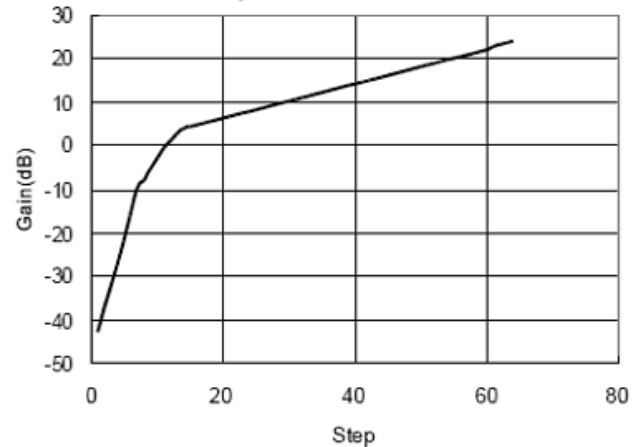
18. Gain Step
