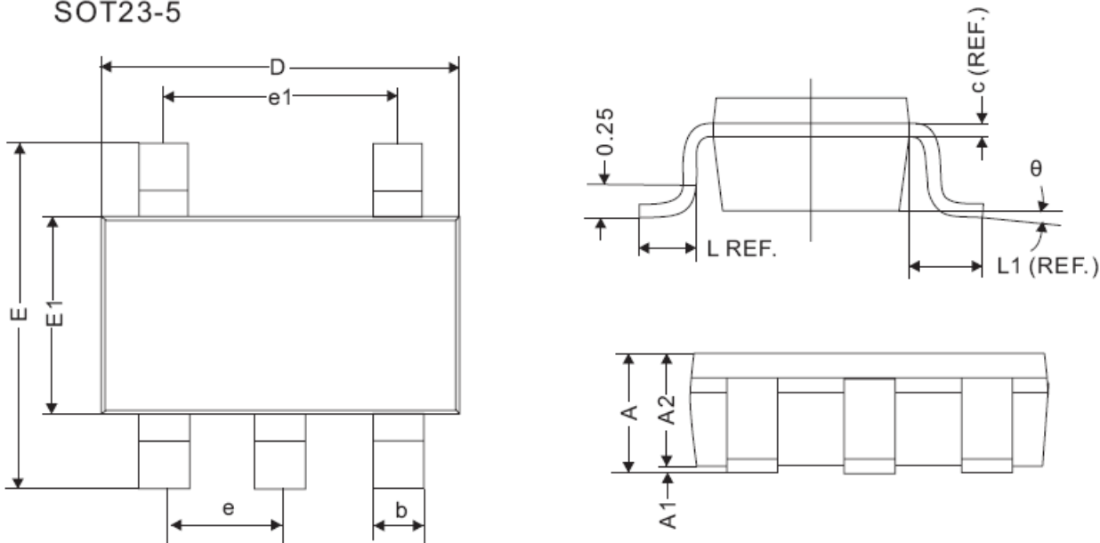
SOT23-5
