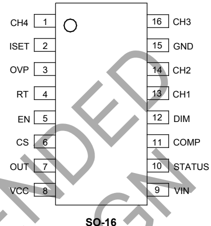
SO-16
