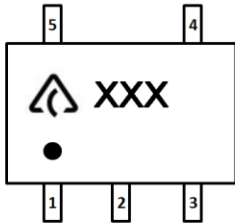
SOT25
