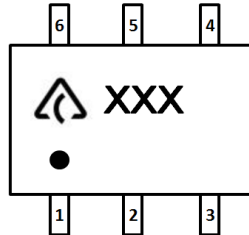
SOT26
