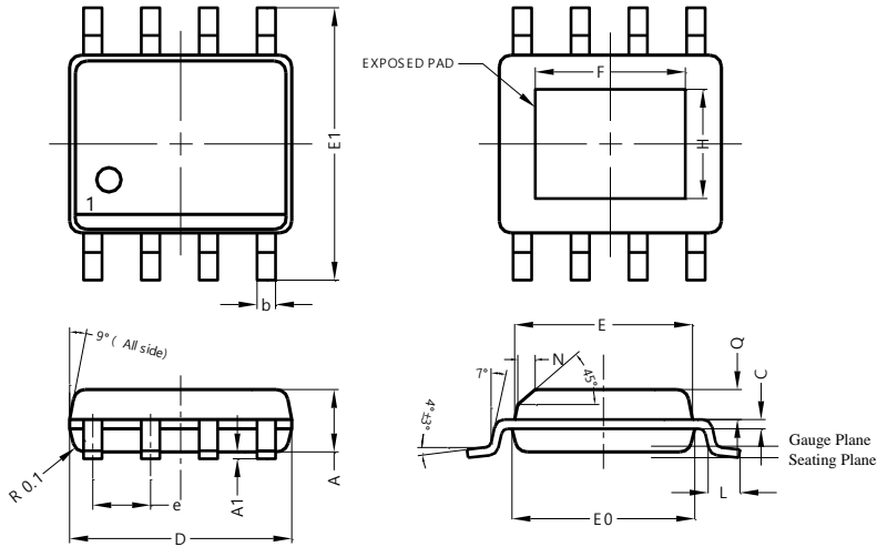
SO-8EP
