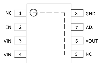
PSOP-8
