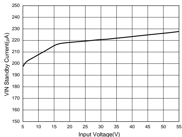
VIN Quiescent Current vs. Input Voltage
