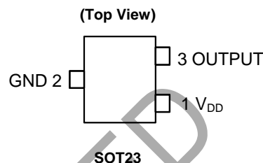
SOT23
