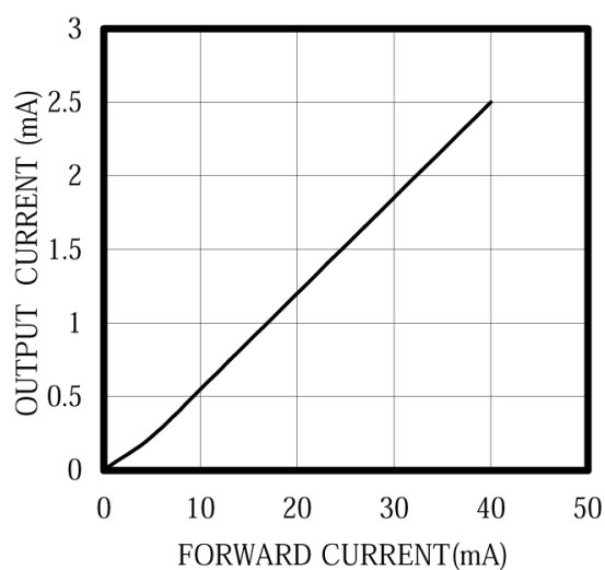
I_F VS I_o V_{CE}=10V
