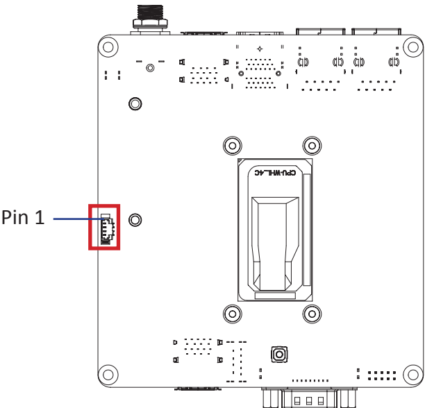
CPU FAN connector
