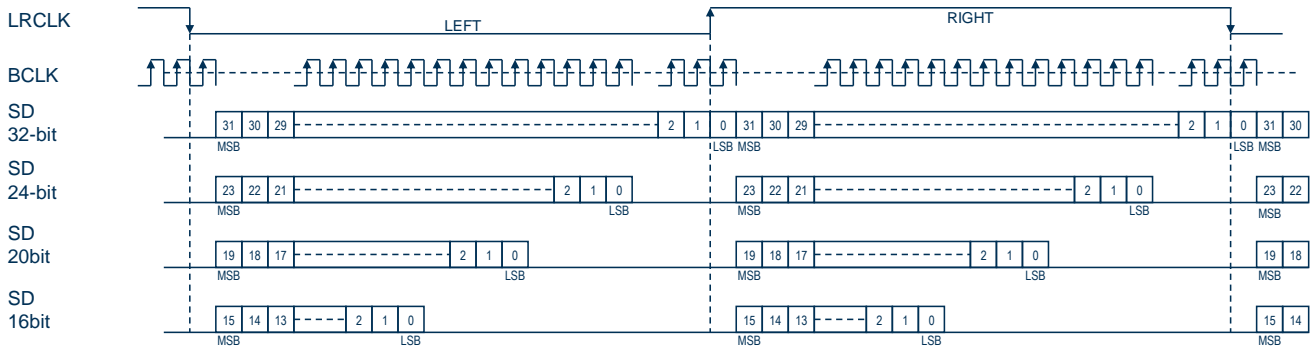
I2S FORMAT
