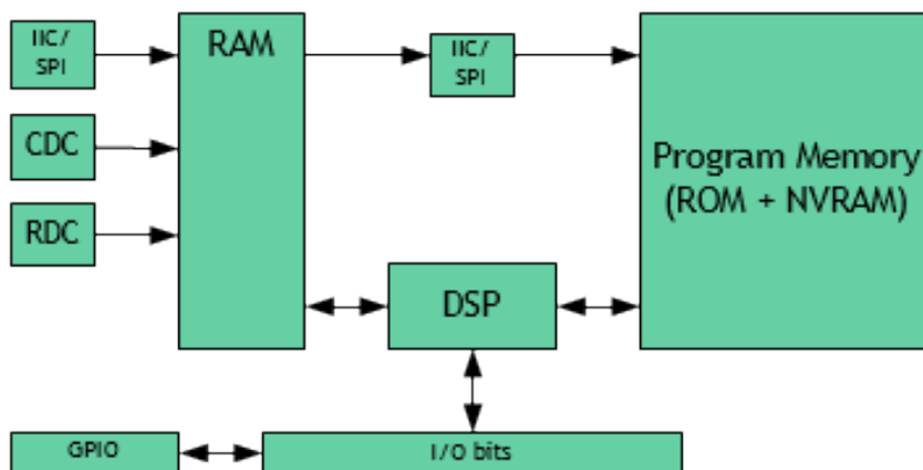
Figure 35: DSP Enabling
