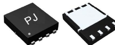
DFN5060-8L
