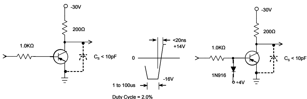
Fig. 1. Turn-On Time
