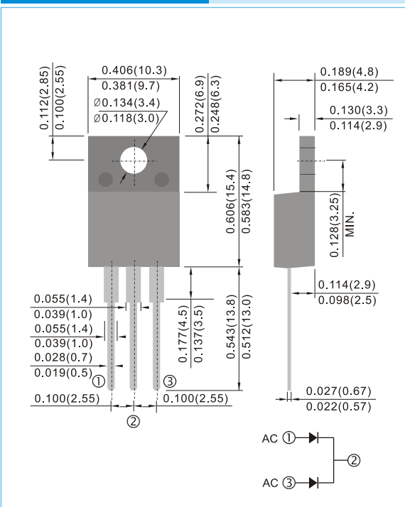
ITO-220AB
