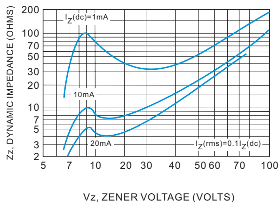
Fig.5 Zener impedance v.s. zener voltage
