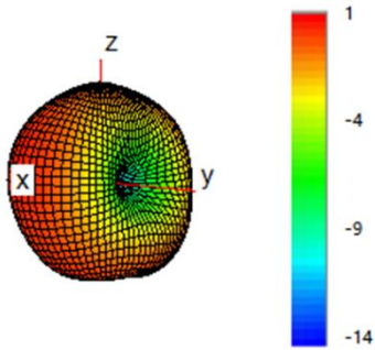
790 MHz
