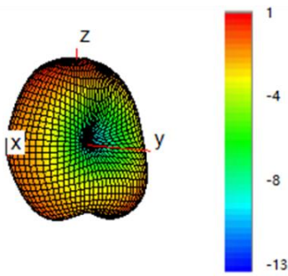
880 MHz
