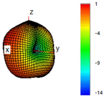
820 MHz
