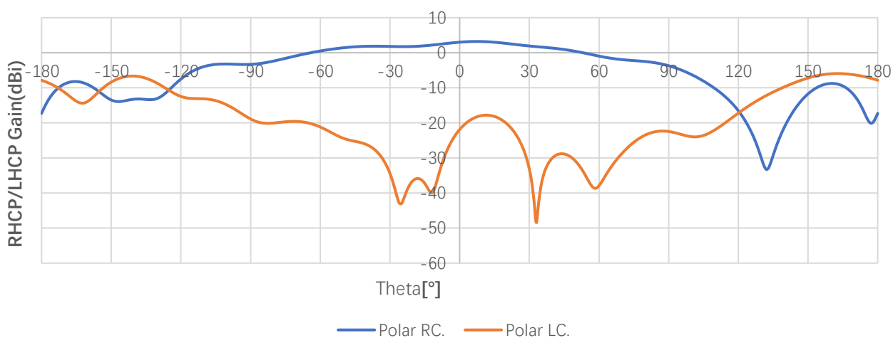
RHCP and LHCP 1602MHz(Phi=90 deg)
