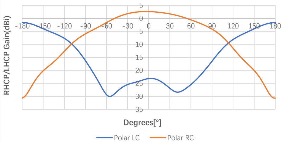
RHCP and LHCP 1561MHz(phi=90deg)
