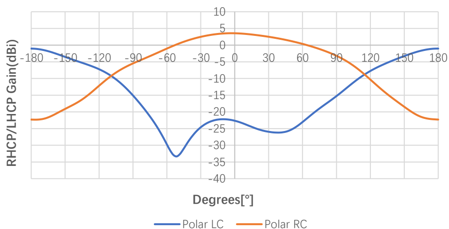
RHCP and LHCP 1575MHz(phi=90deg)
