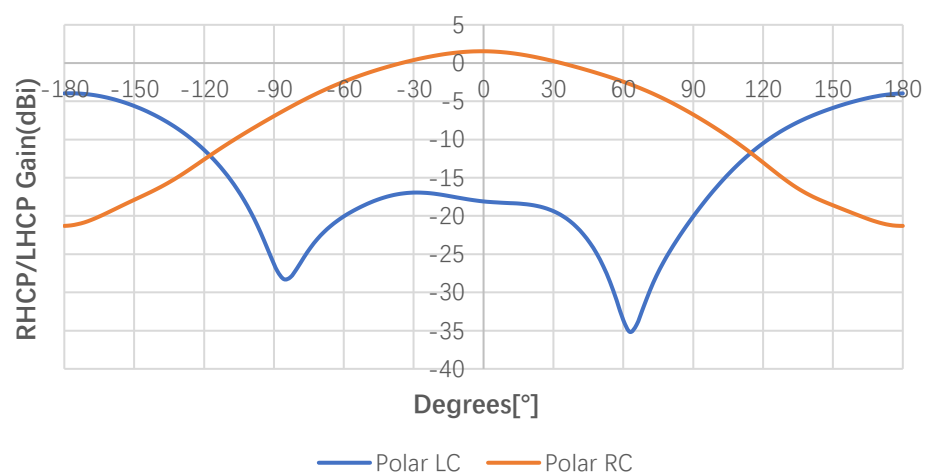
RHCP and LHCP 1602MHz(phi=0deg)
