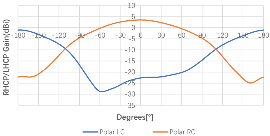
RHCP and LHCP 1575MHz(phi=0deg)
