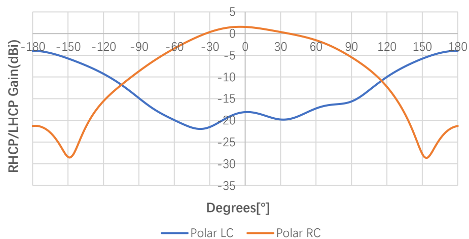
RHCP and LHCP 1602MHz(phi=90deg)
