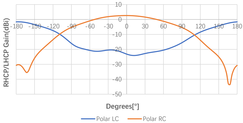
RHCP and LHCP 1561MHz(phi=0deg)
