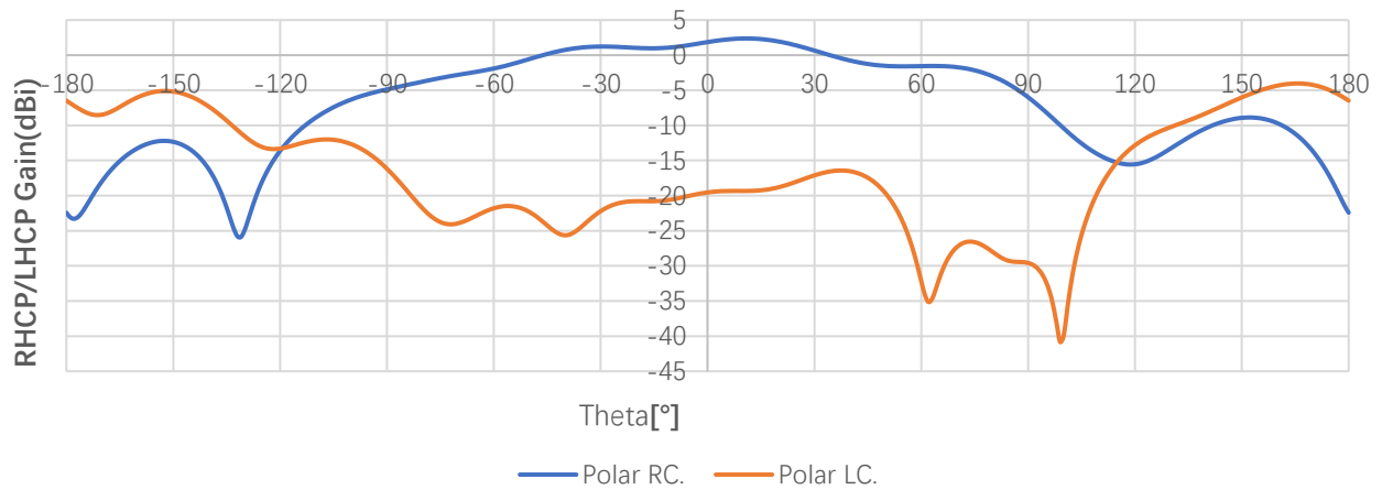
RHCP and LHCP 1561MHz(Phi=90 deg)
