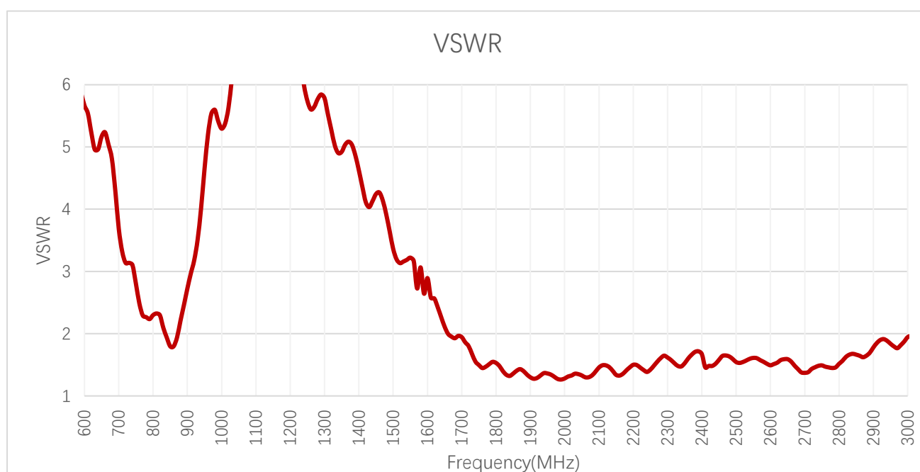
VSWR - 4G
