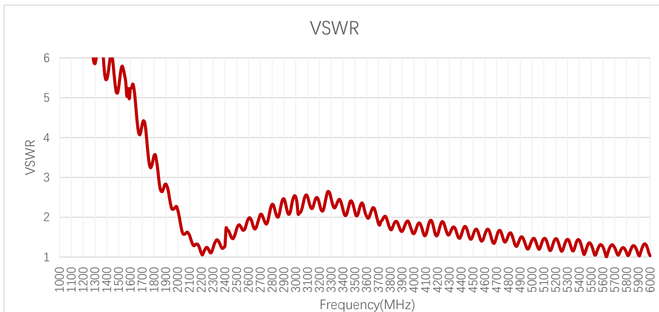
VSWR - Wi-Fi
