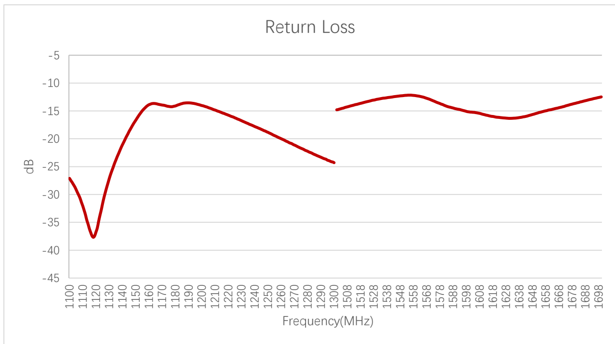
Return Loss(dB)-GNSS
