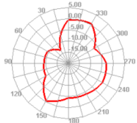
2100.000MHz E1
