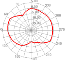
2650.000MHz E2
