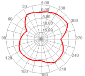
2650.000MHz
