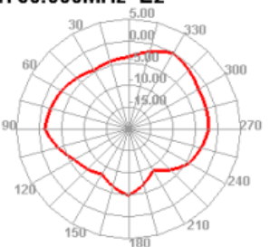
1750.000MHz E2
