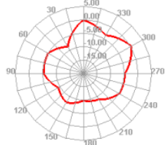
2650.000MHz E1
