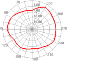
2650.000MHz E2
