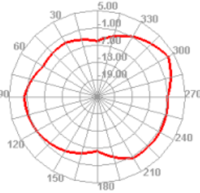
1700.000MHz E2
