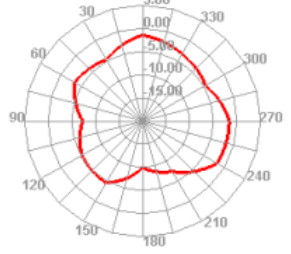
2400.000MHz E2
