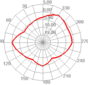
1700.000MHz E2
