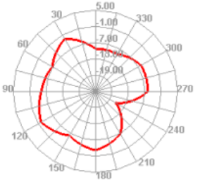
2100.000MHz E2
