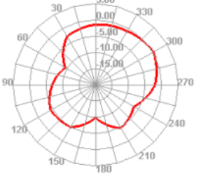
2650.000MHz H
