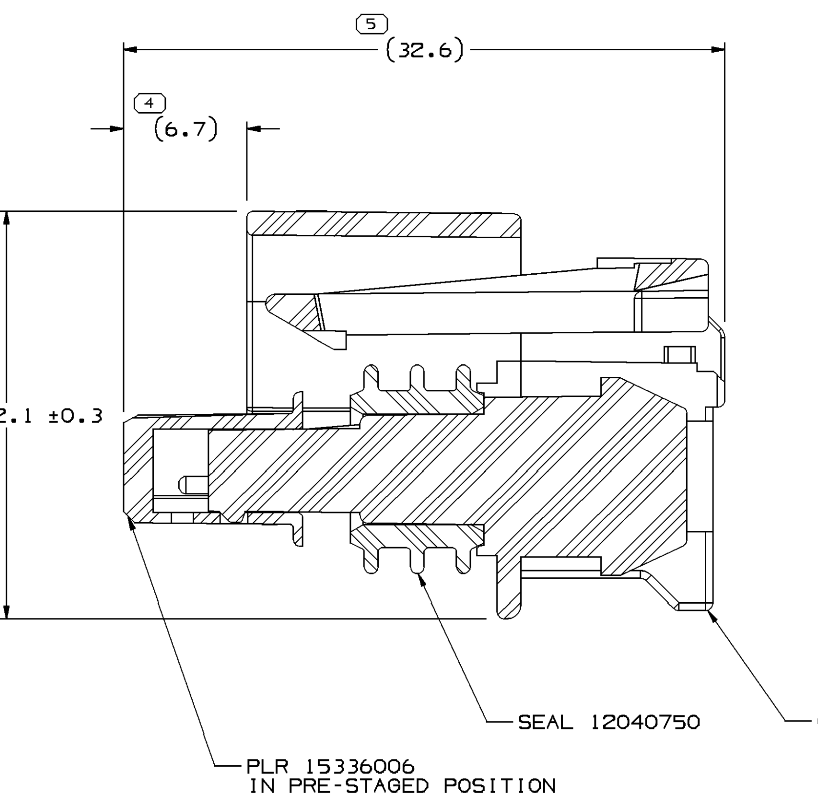
SECTION A-A
