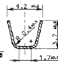
SEZ. B-B PER CONTATTO VERSIONE B
