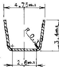
SEZ. C-C
