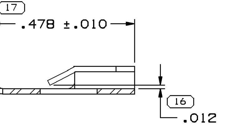
SECTION A-A TYPE 402
