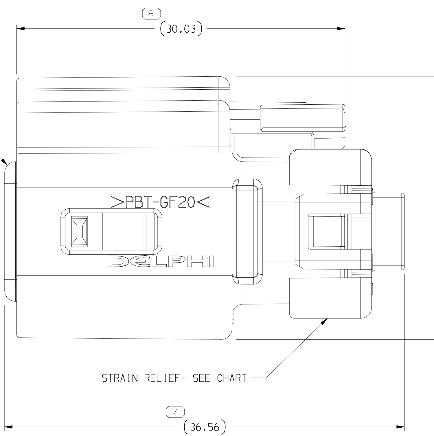
TYPE 101
