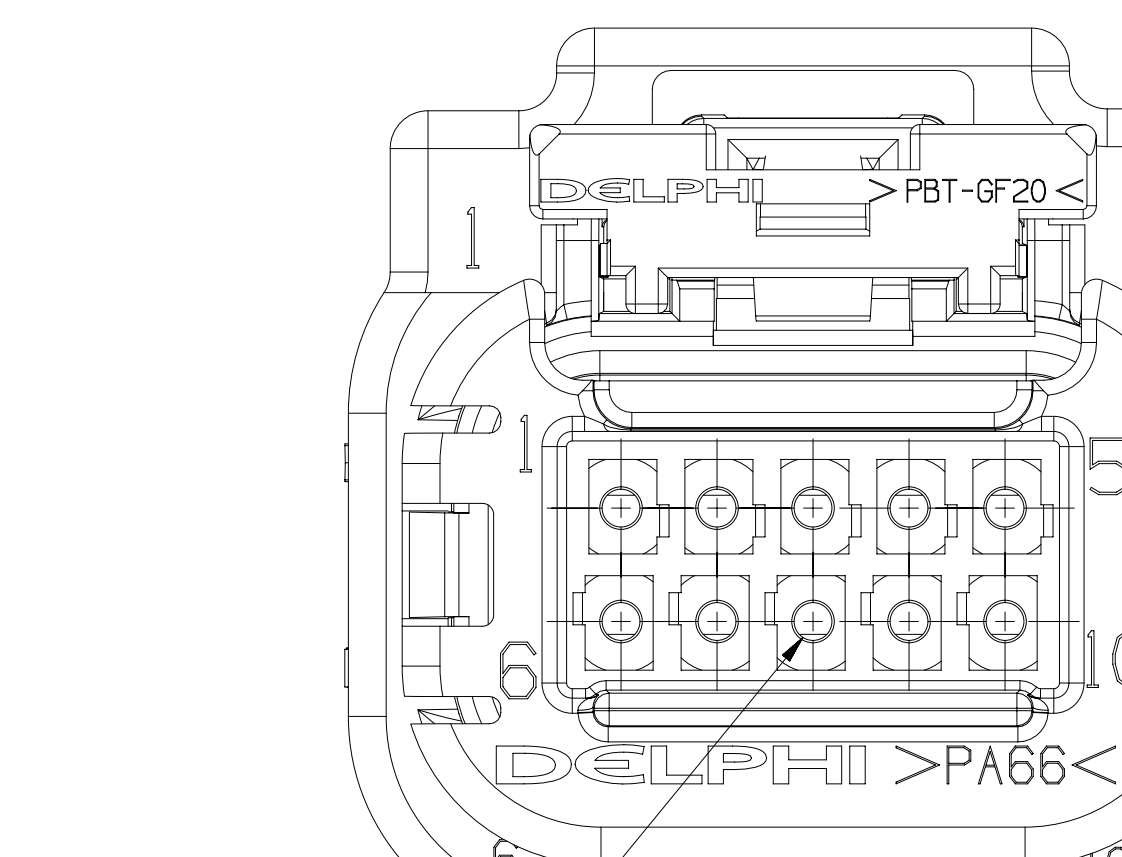
TYPE 101
