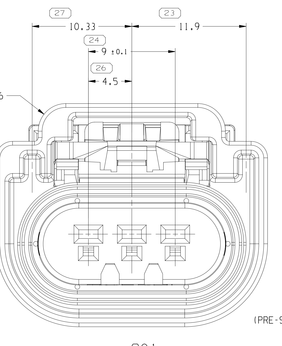
TYPE 201
