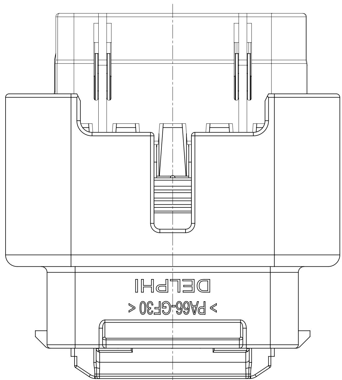
C.P.A & T.P.A IN PRE LOCK POSITION
