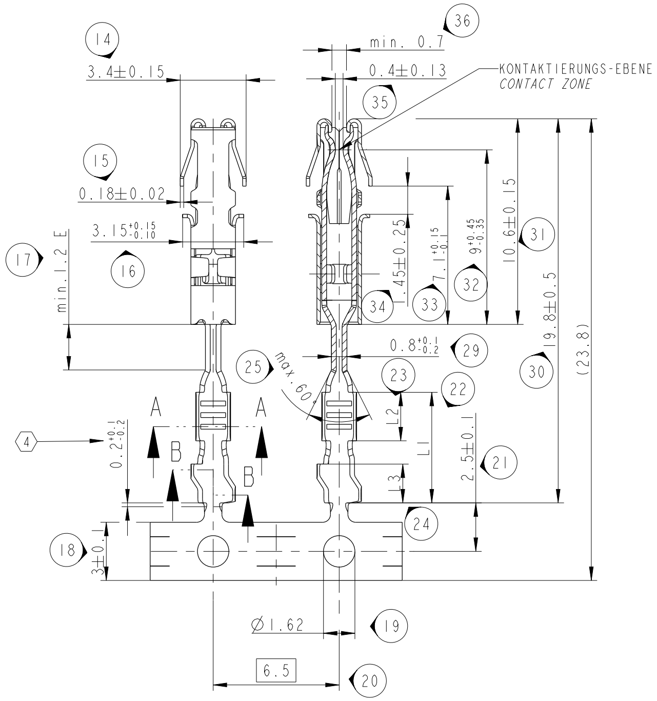
BILD 1.DCK 1.5 NWD CRIMPBEREICH (>0.22-0.35)mm 2 -DELPHI TEILE-NR. F843410; OBERFLÄCHE FEUERVERZINNT PICTURE 1. DCK 1.5 NWP FOR CRIMP RANGE (>0.22-0.35)mm 2 -DELPHI PART-NO. F843410; CONTACT FINISH HOT DIP TIN
