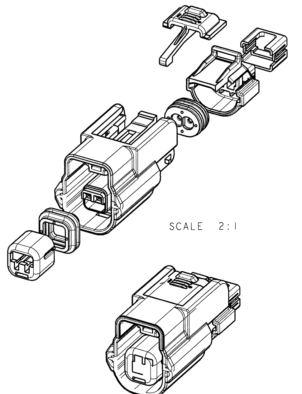
SCALE 2:1
