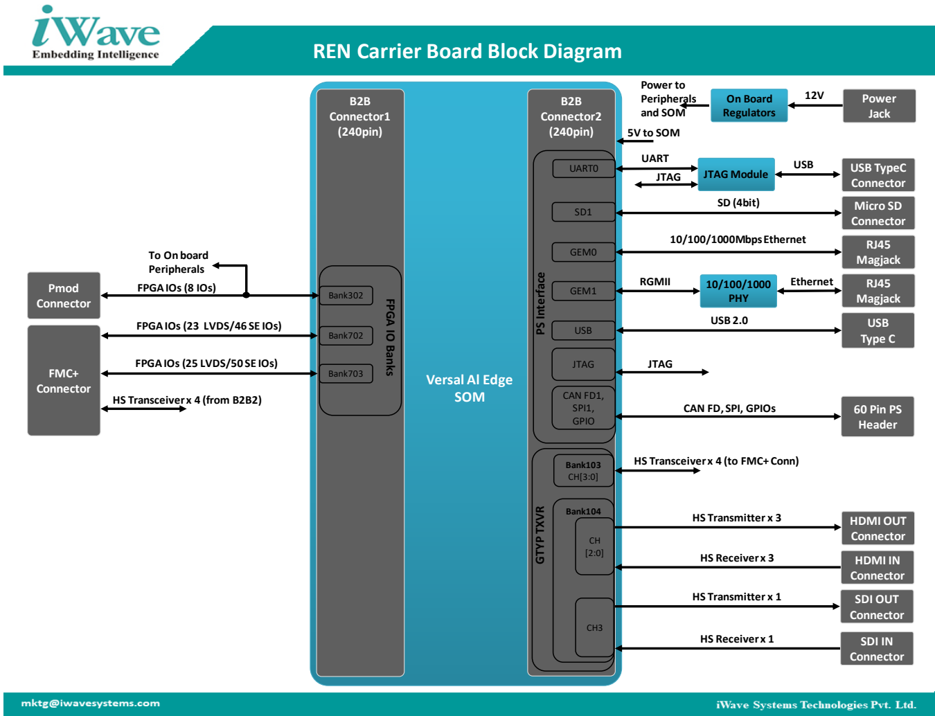
Figure 1: Versal AI Edge SOM Carrier Board Block Diagram
