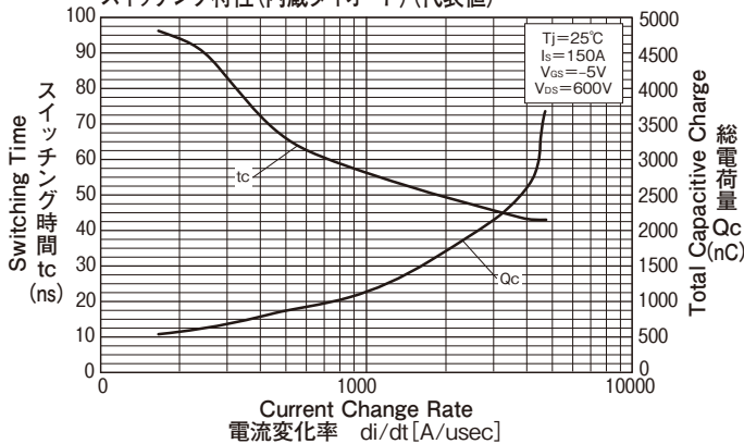
Switching Characteristics (Integrated Diode) (Typical) スイッチング特性 (内蔵ダイオード) (代表値)
