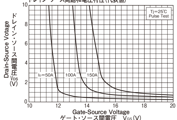
Drain-Source Saturation Voltage Characteristics (Typical) ドレイン・ソース間飽和電圧特性 (代表値)
