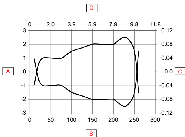
Fig. 4 PD30ETBS25BPxxIO
