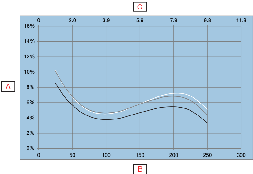
Fig. 6 PD30CTBR20BPxxIO
