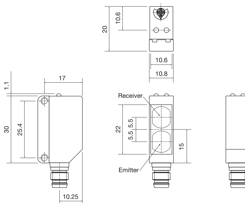
Fig. 5 Plug
