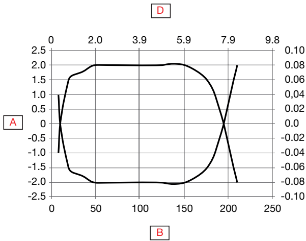
Fig. 4 PD30CTBR20BPxxIO
