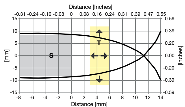
Fig. 4 M18 Non-flush
