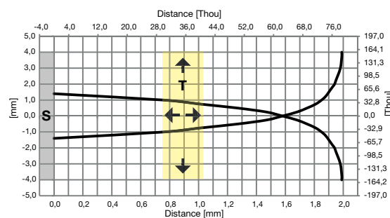
Fig. 2 Flush, 2mm
