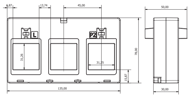
Fig. 17 TCD3X (mm)
